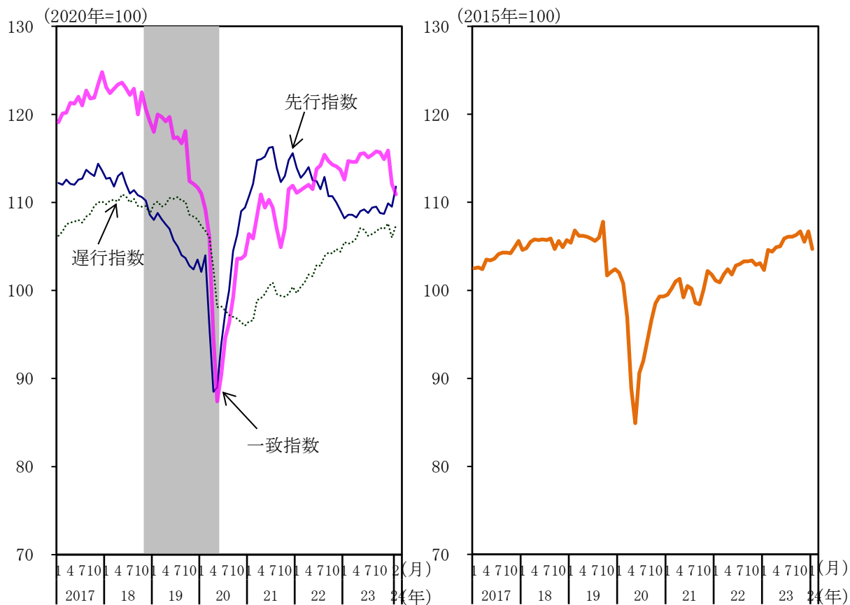
CIの推移
