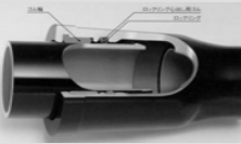
耐震管(継手)の例
