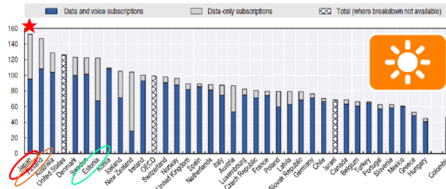
■ モバイルブロードバンド普及率（100人あたり、2016年）
