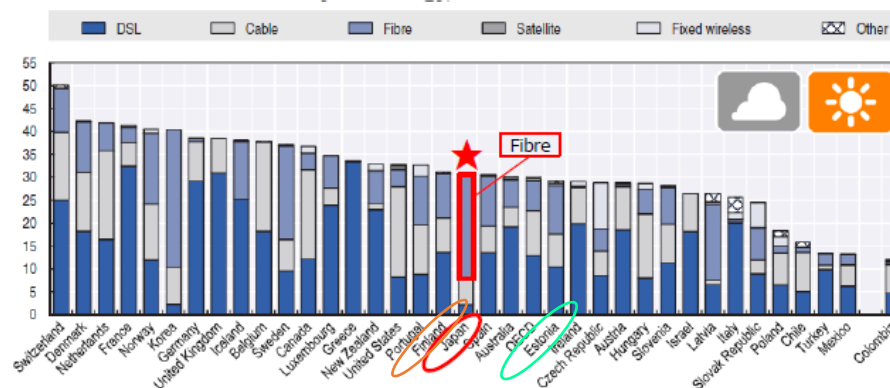
■ 固定ブロードバンド普及率（100人あたり、2016年）
