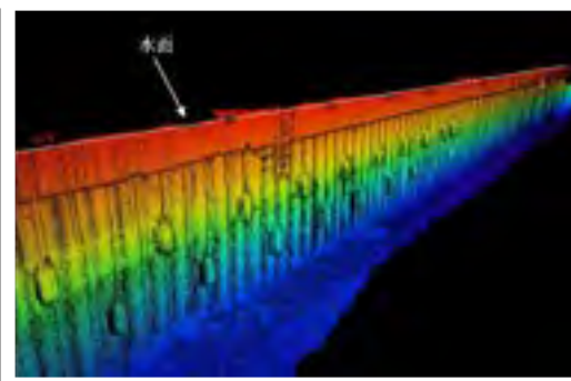
測量結果
