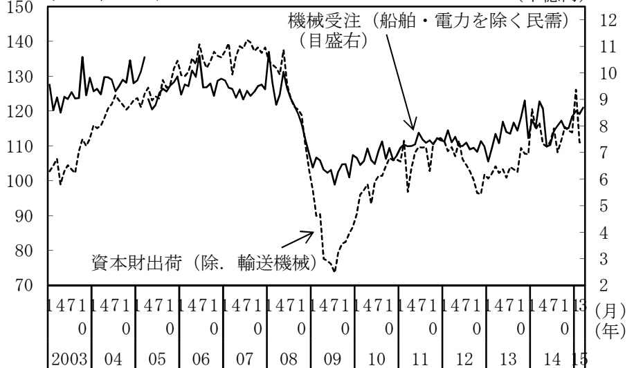
(2010年=100) 資本財出荷指数と機械受注 (千億円)
